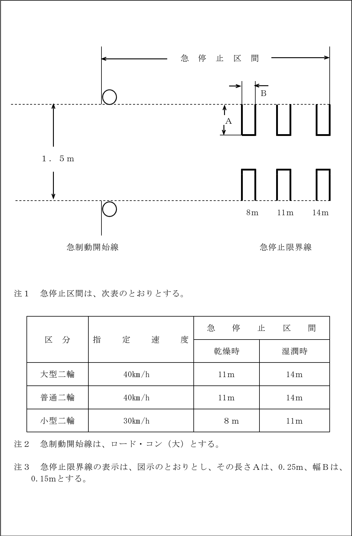
指定速度からの急停止コース（設置例）
